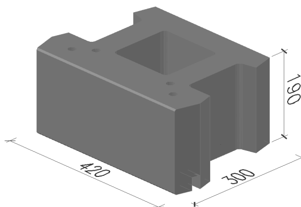
Rys. 1. Bloczek betonowy
